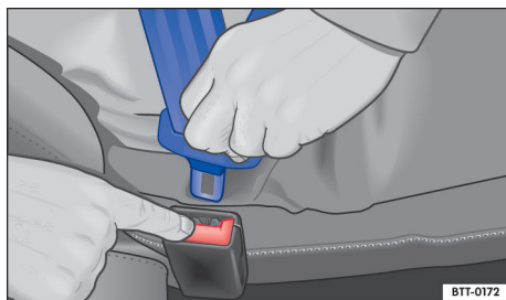
图 28 从插口上松开安全带锁舌
