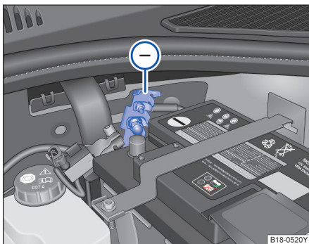
图 129 身上的负极（接地点）
