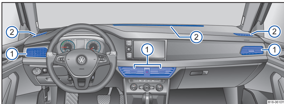
图 82 前部通风口
