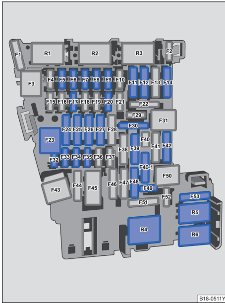
图 124 保险丝位置示意图
