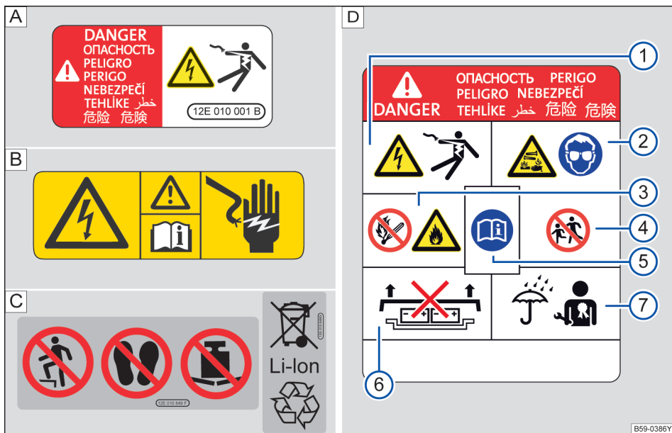
图 108 警告牌（示意图）：A 高压组件，B 高压电普通警告牌，C、D 高压蓄电池上的警告牌
