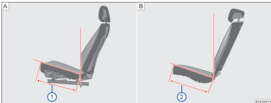
图 63 座椅坐垫深
