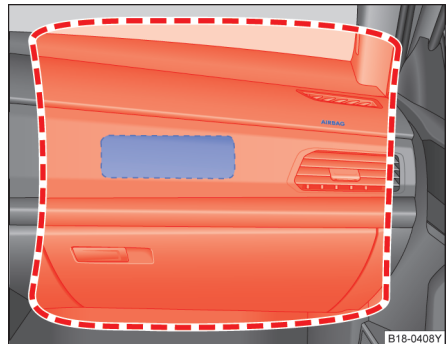
图 33 副驾驶员前部安全气囊的安装位置和膨胀范围
